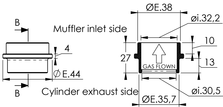
B-B section 1 : 2 - SCALE
