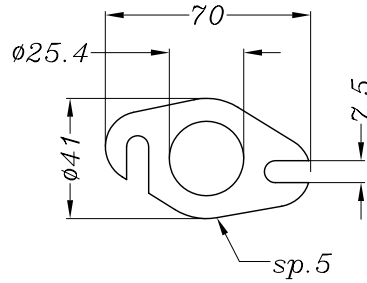
Vista da "A" Flangia tipo "96A"
