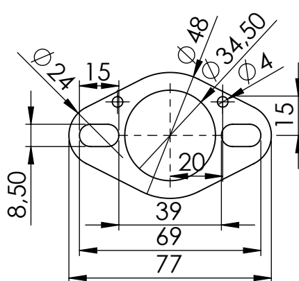
S.s. flange sp.5mm Cod.206443
