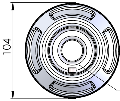
dB-killer Ø22 Cod.303430803
