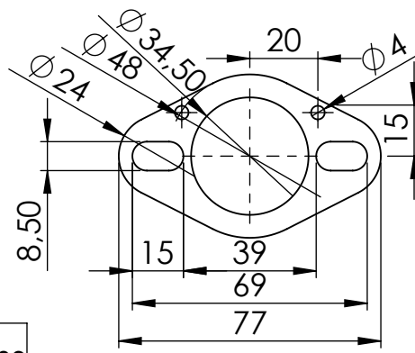
"S.S. flange" Cod.206443
