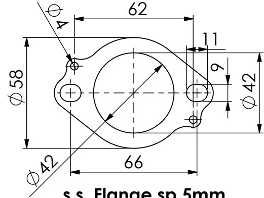
s.s. Flange sp.5mm cod.207024
