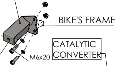
3x Knurled collar nut M6 Cod.200333
