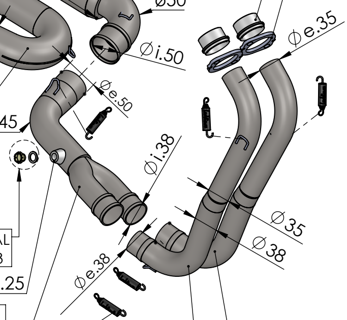
2x Flange cod.204569
