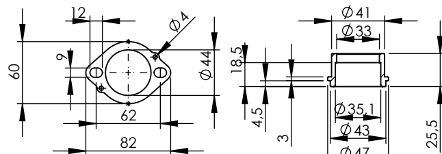
S.s Flange 112A cod.204569 Sp.5mm
