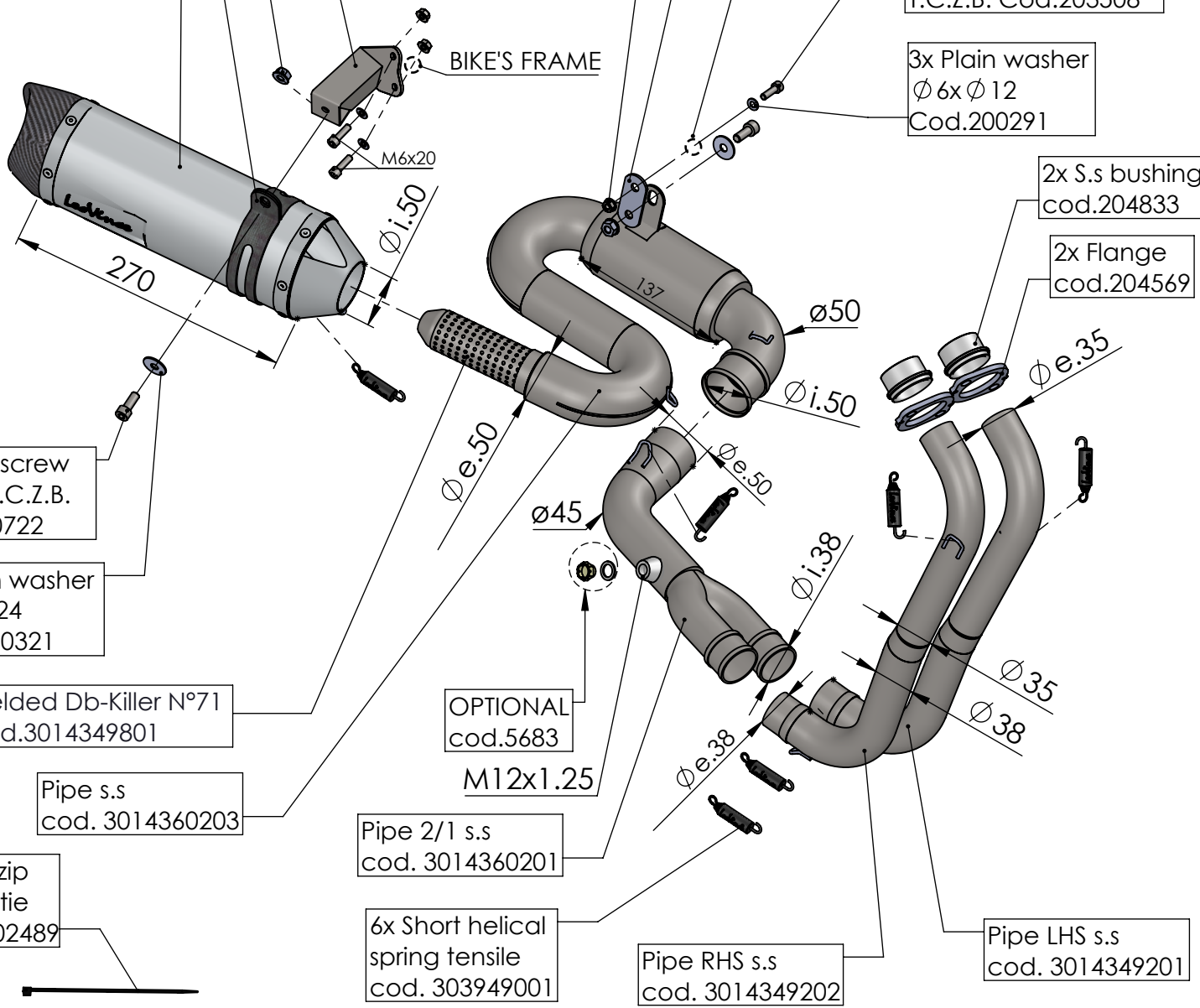
3x Allen screw M6X20 T.C.Z.B. Cod.203508
