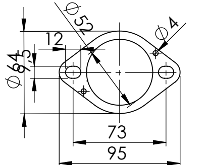
Flange s.s. sp.5mm cod.206423
