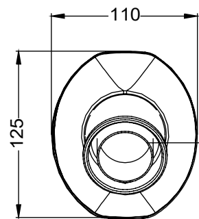
VISTA DA "A"
