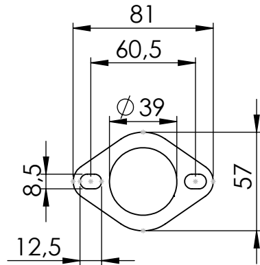
S.S. Flange 25B P/N 200560
