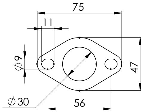
S.S. Flange - 45D P/N 204680
