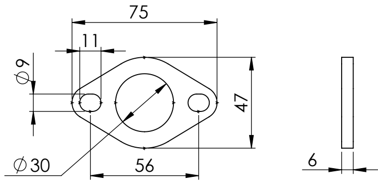
S.S. Flange - 45D P/N 204680
