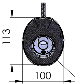
dB-Killer n°62 kit P/N 3014259801R
