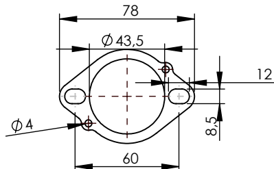
S.S. Flange 46D P/N 204448R
