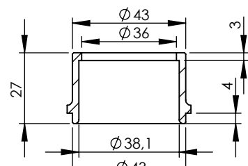
S.S. Bushing P/N 204870R
