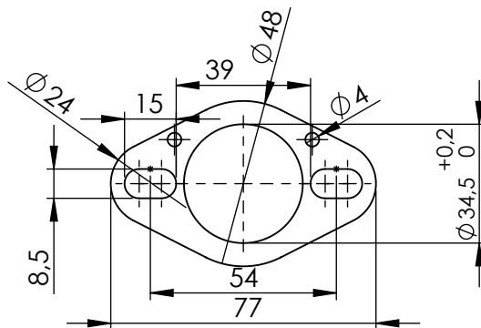
S.s. Flange Cod.206443R
