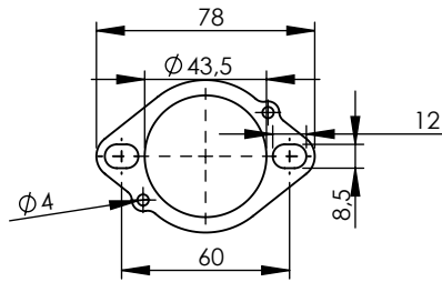
s.s. flange "46D" sp.5mm cod.204448R
